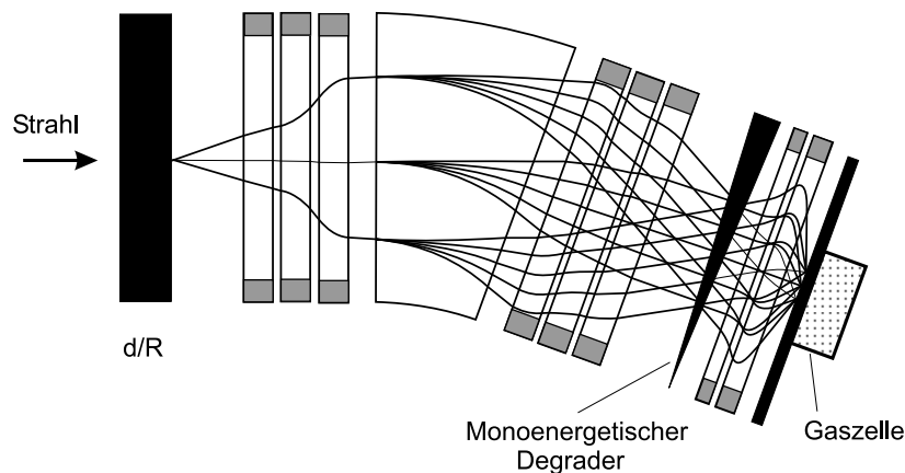
Abbildung 5.8: System zur Reichweitefokussierung bestehend aus einem ersten dicken Degradier, einer Dipolstufe, dem keilförmigen zweiten Degradier und einem Quadrupoldelement um einen schmalen Strahldurchmesser im Implantationsvolumen zu erhalten.
