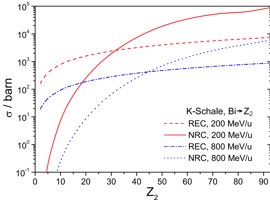
Abbildung 2.7: Einfangquerschnitt direkt in die leere K-Schale von Bismutationen als Funktion von Z_2 aufgeteilt nach Anteilen des REC (nicht relativistische Dipolapproximation) und NRC (Eikonapproximation), Werte nach GLOBAL [SSM98].
