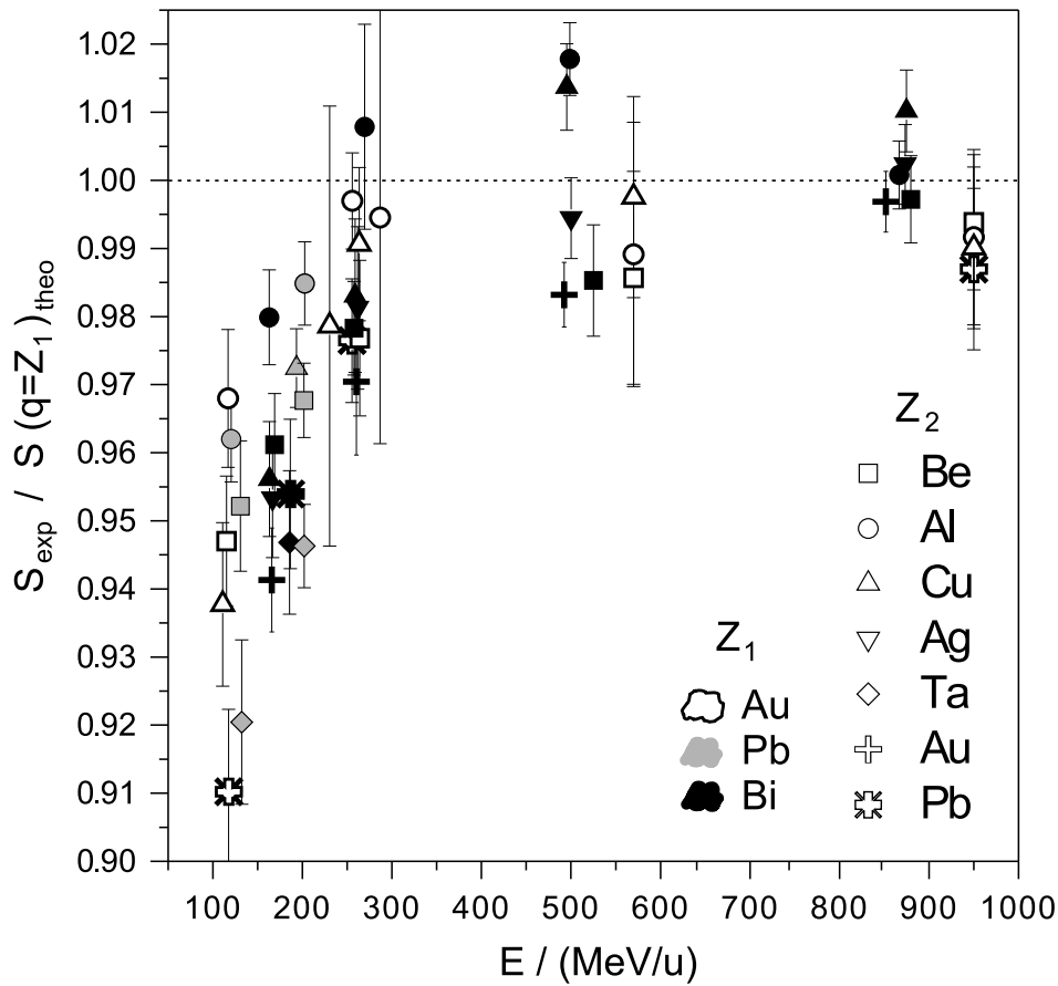
Abbildungung 4.6: Experimentelle Stopping-Power für ^{197}\text{Au} -, ^{208}\text{Pb} - und ^{209}\text{Bi} -Projektilen in verschiedenen Targetmaterialien normiert durch die entsprechenden Werte der LS-Theorie. Die theoretische Rechnung wurde für nackte Projektilen gemacht.
